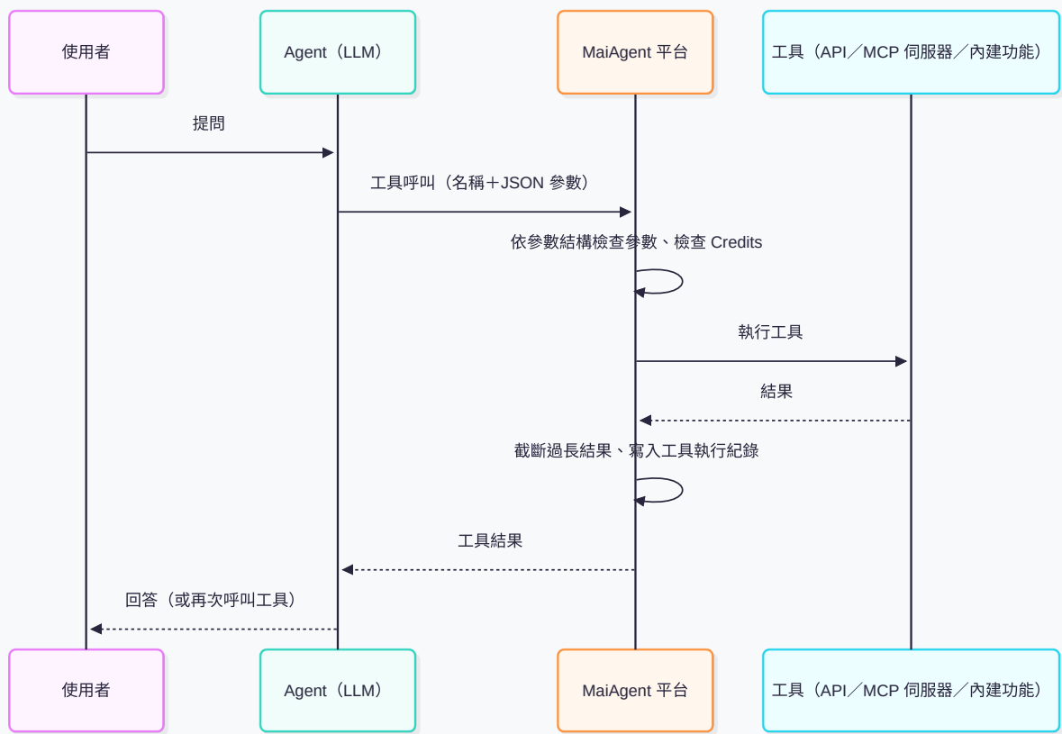
Mermaid 圖表
